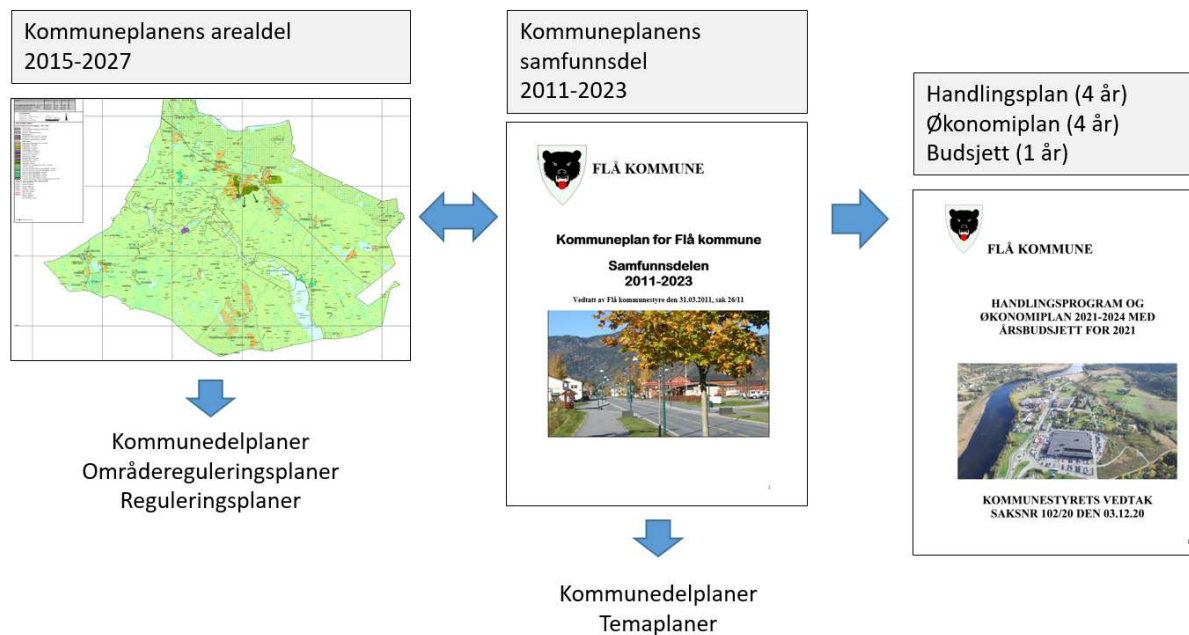
Figur 1-1 Kommunens plansystem.
