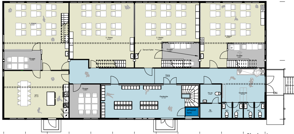
Planløsning 1 etg.
